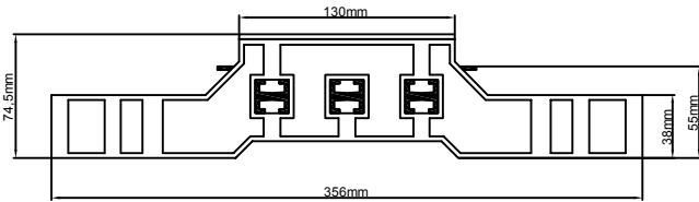
Busbar Type 1 250A
