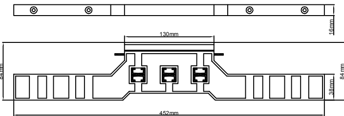
Busbar Type 3 250A
