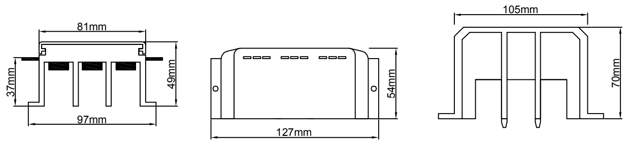
Busbar Type 0 250A
